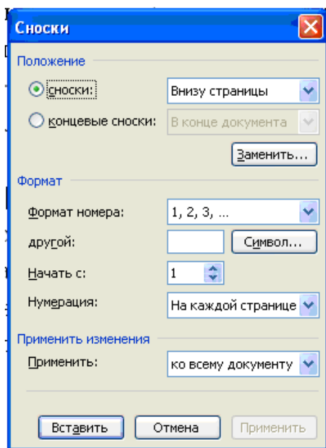
Рисунок 2 – Параметры сносок
