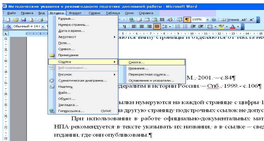
Рисунок 1 – Вставка сноски
